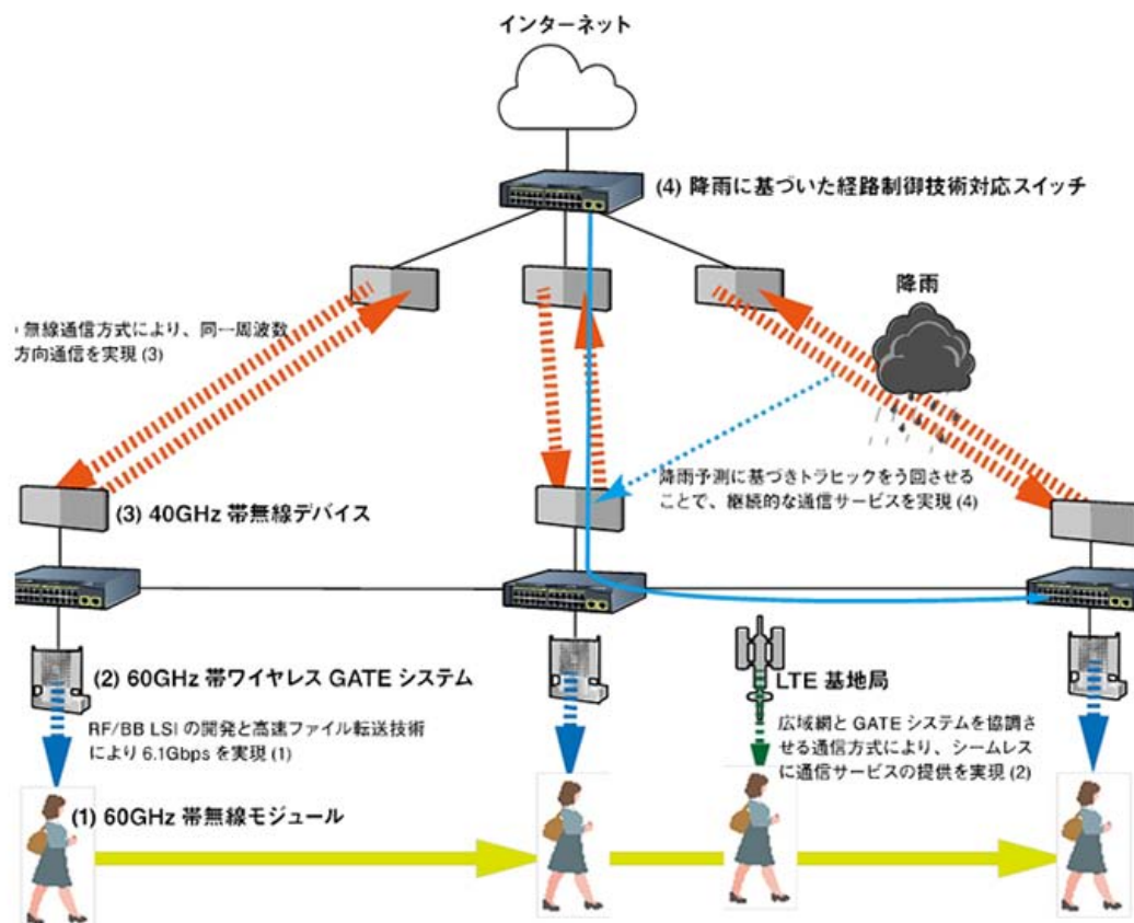
図1. 共同研究開発したシステムの全体像
