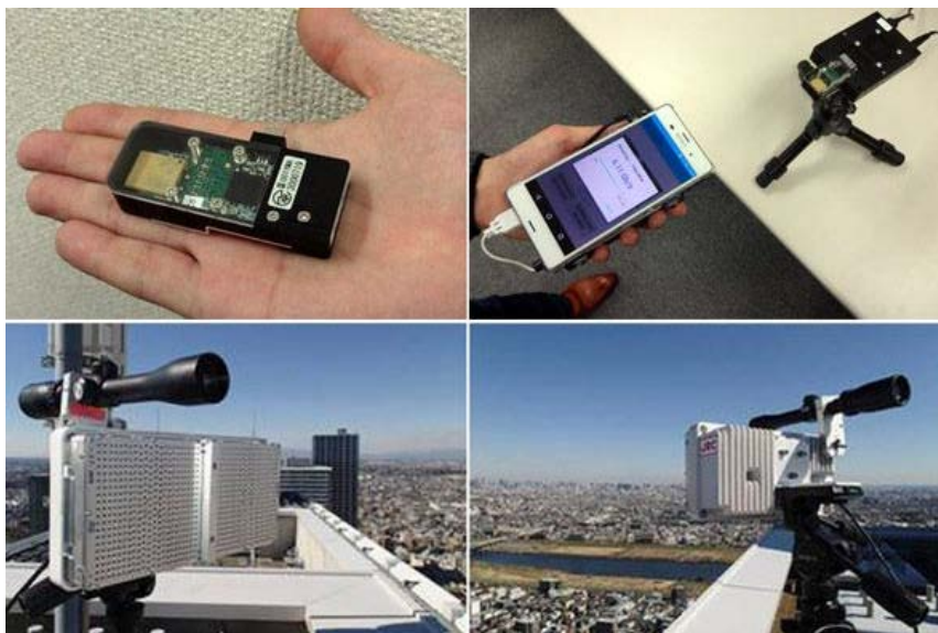
60GHz帯通信モジュールによる6.1Gbpsのモバイル通信（上）、アクセスポイントの40GHz帯通信の連携試験（下）
